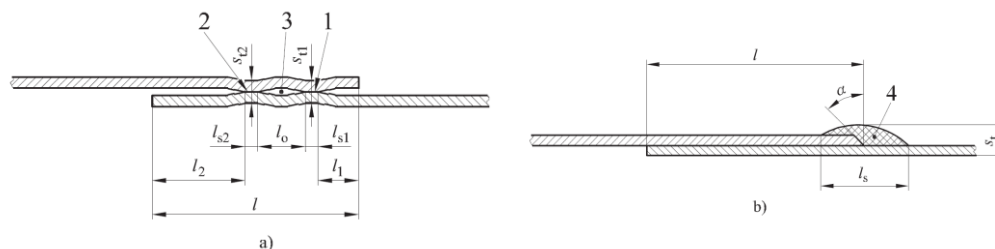
Figura 1 – Giunto a doppia saldatura (a) ed a cordone sovrapposto (b)
