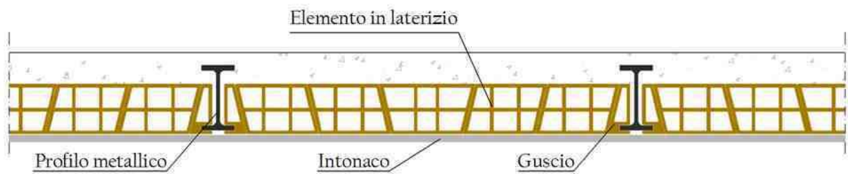
Disegno n°3 - Schematizzazione dell'andamento della sezione della Tipologia Solaio 1.
