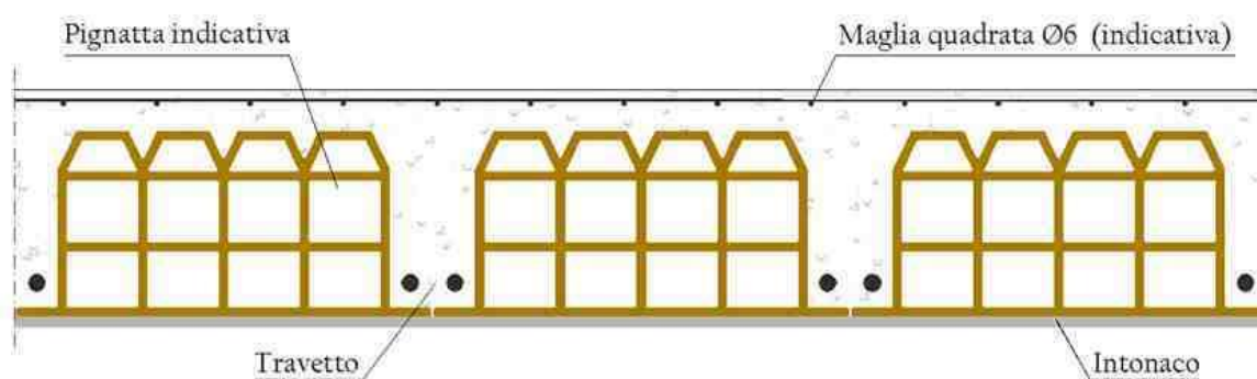
Disegno n°4 - Schematizzazione dell'andamento della sezione della Tipologia Solaio 2.
